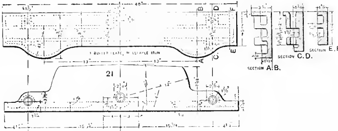
Figs. 1380-1384. Buffer Plate, Malleable Iron.
